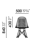
Wire Chair DKR, vier poten draadonderstel met dwarsverbindingen
