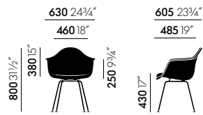
Eames Plastic Armchair DAX, vierpots-staalbuisonderstel volledig bekleed
