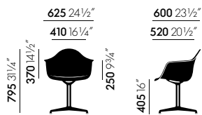
Eames Plastic Armchair DAL, voet persgietaluminium gepolijst
