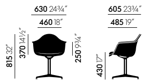
Eames Plastic Armchair DAL, voet persgietaluminium gepolijst volledig bekleed
