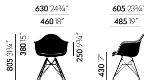
Eames Plastic Armchair DAR, draadonderstel met schoren volledig bekleed
