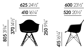
Eames Plastic Armchair DAR, draadonderstel met schoren
