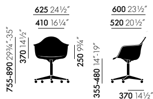
Eames Plastic Armchair PACC, draaibare stoel op zwenkwheels
