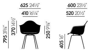
Eames Plastic Armchair DAX, vierpots-staalbuisonderstel
